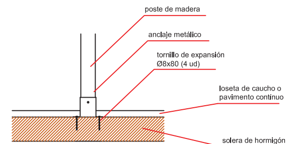
DETALLE DE ANCLAJE
