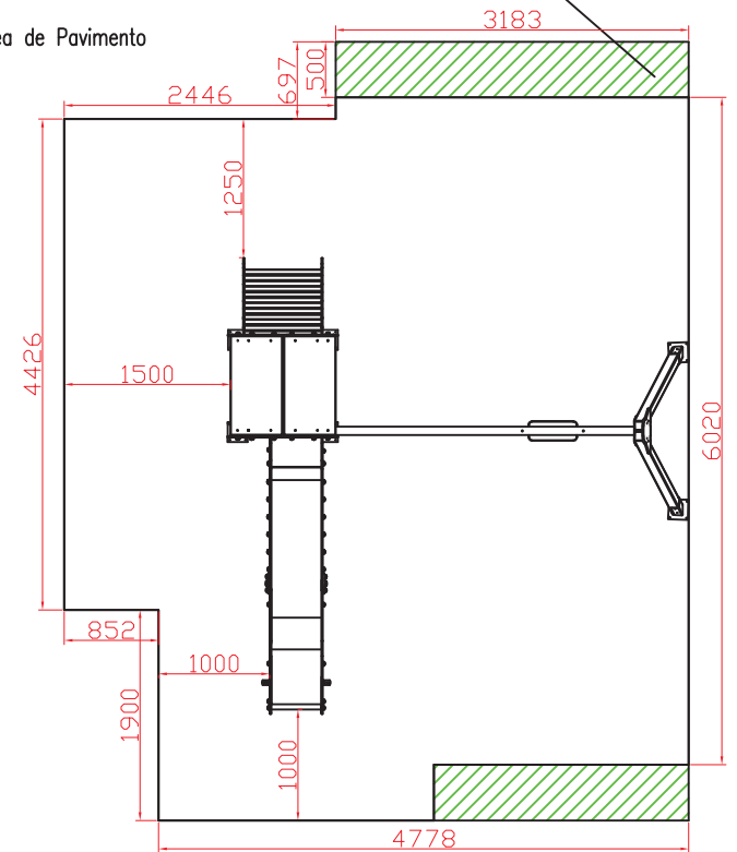
AREA DE SEGURIDAD AREA=33,46 m2
