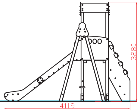
PERFIL IZQUIERDO
