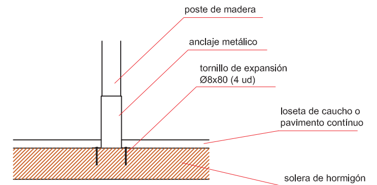
DETALLE DE ANCLAJE E:2/1
