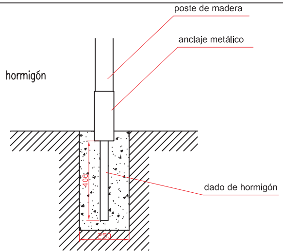
DETALLE DE CIMENTACIÓN E:2/1
