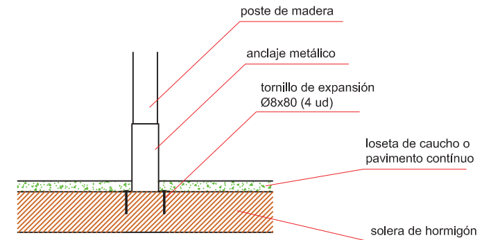
DETALLE DE ANCLAJE ATORNILLADO
