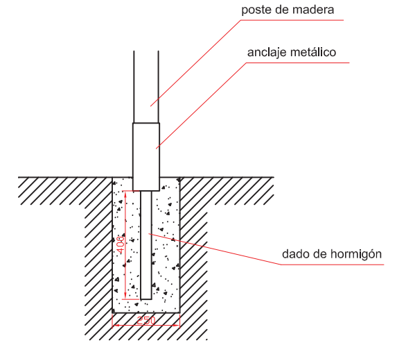
DETALLE DE CIMENTACIÓN
