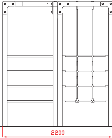
Perfil Derecho
