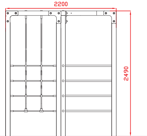
Perfil Izquierdo
