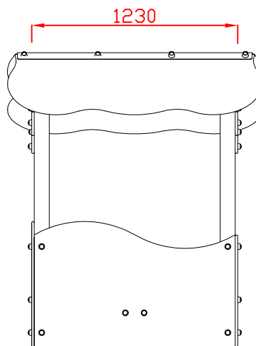
PERFIL IZQUIERDO
