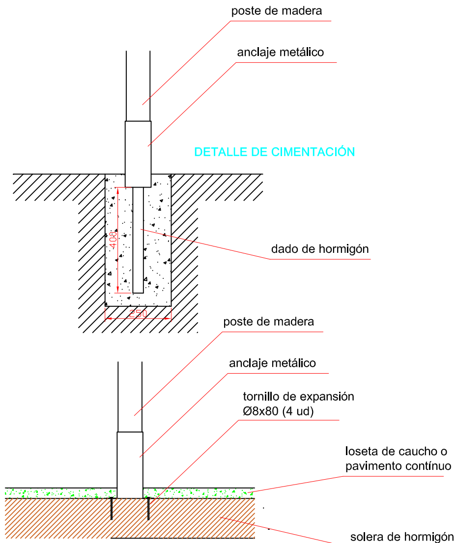
DETALLE DE ANCLAJE ATORNILLADO
