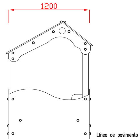
ALZADO POSTERIOR
