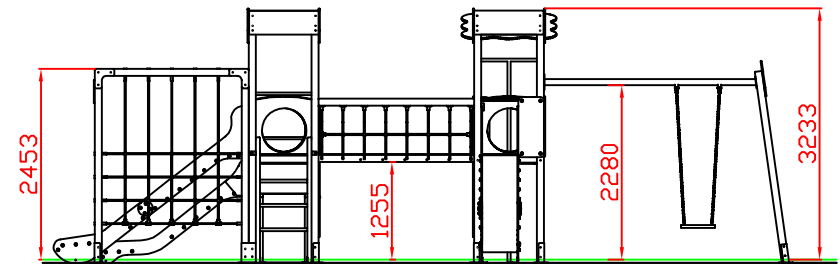
PERFIL DERECHO
