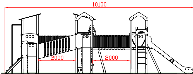
ALZADO
