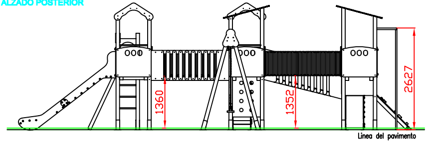
ALZADO POSTERIOR
