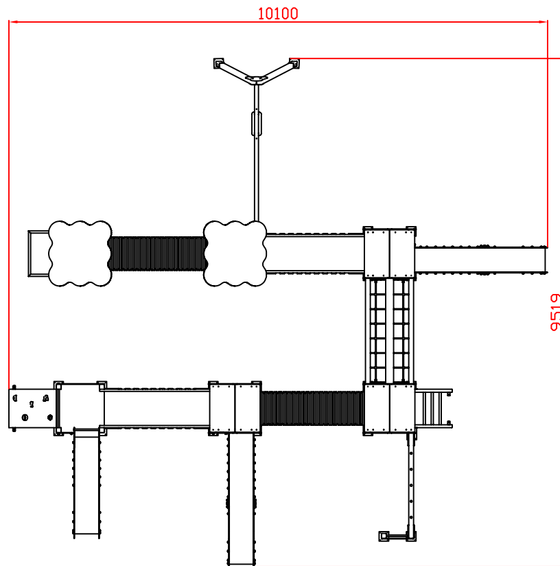
PLANTA
