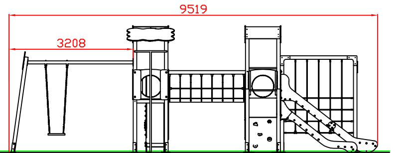
PERFIL IZQUIERDO
