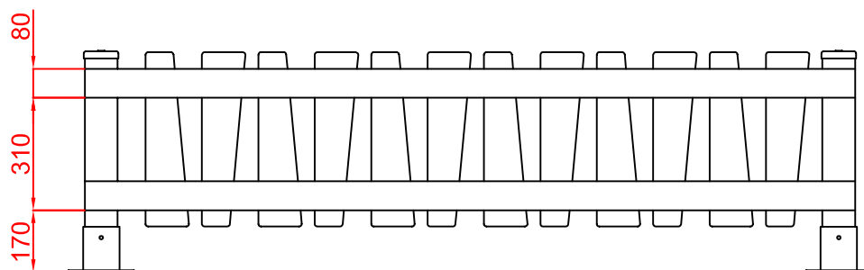
ALZADO POSTERIOR
