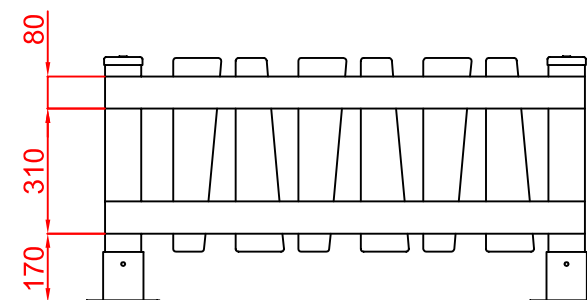
ALZADO POSTERIOR
