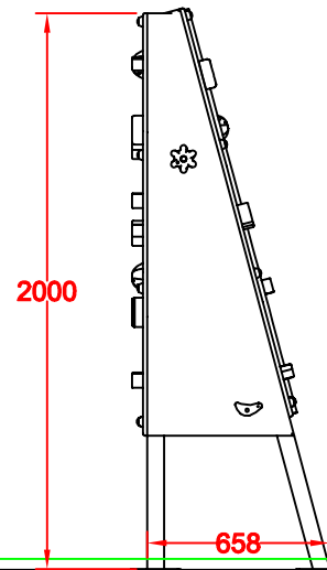
PERFIL IZQUIERDO
