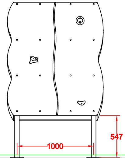
ALZADO POSTERIOR
