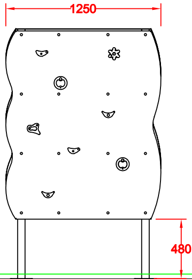
ALZADO
