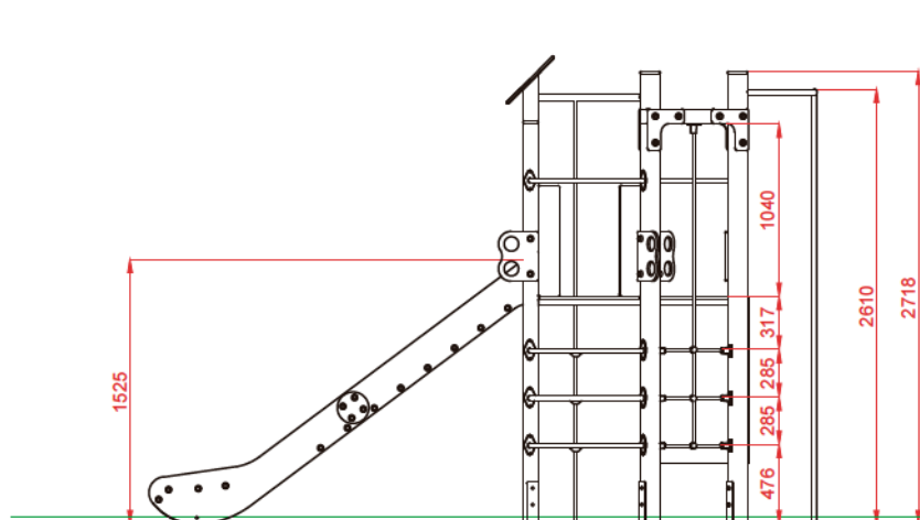
ALZADO
