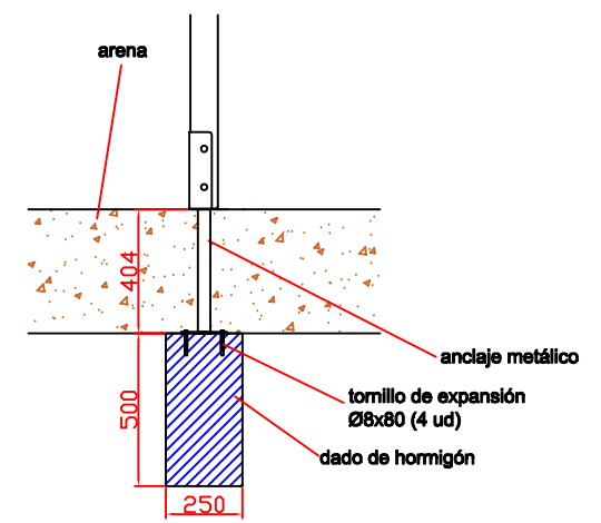
ESQUEMA DE CIMENTACIÓN PARA CASOS EN LOS QUE VA EN ARENERO E2/1
