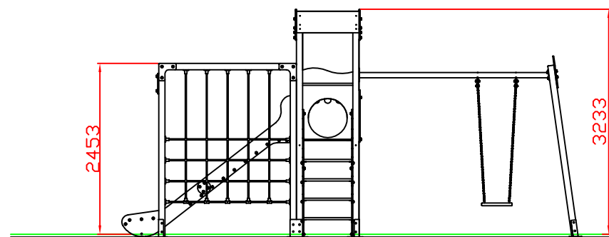
ALZADO
