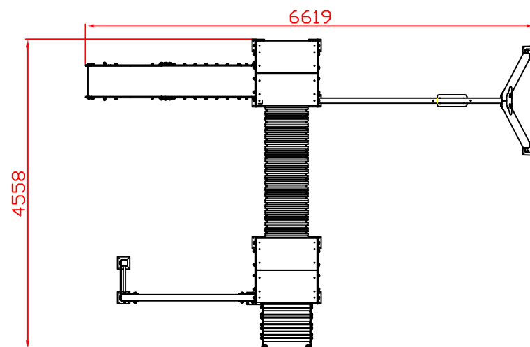
PLANTA
