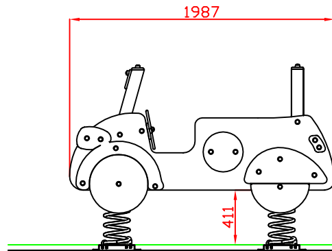
PERFIL DERECHO
