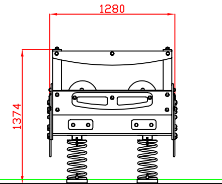
ALZADO
