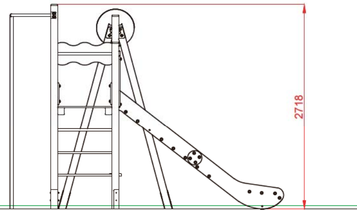
PERFIL IZQUIERDO
