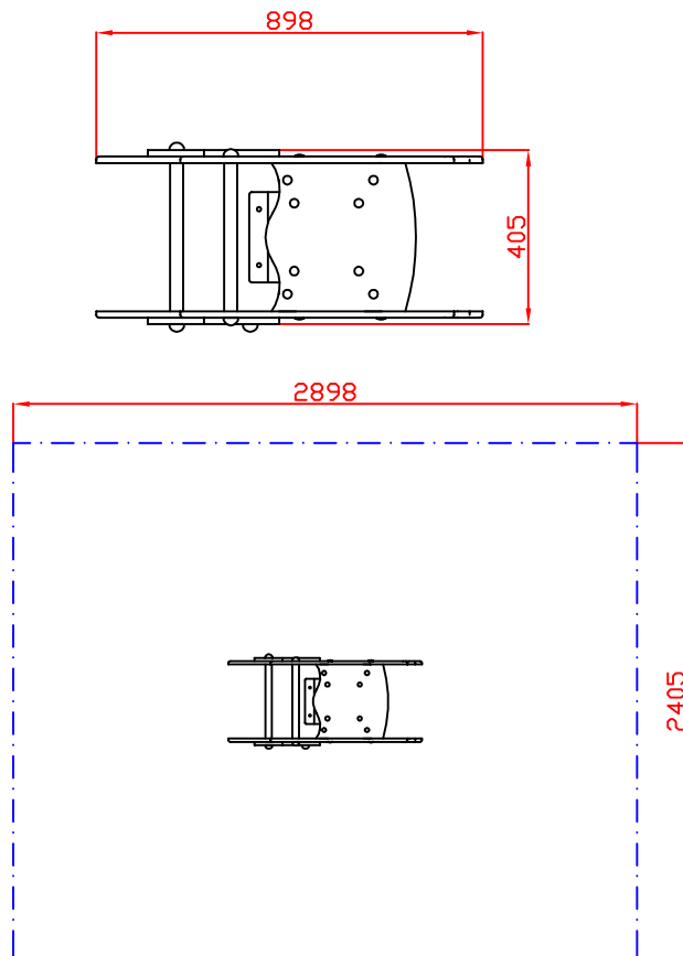
Planta
