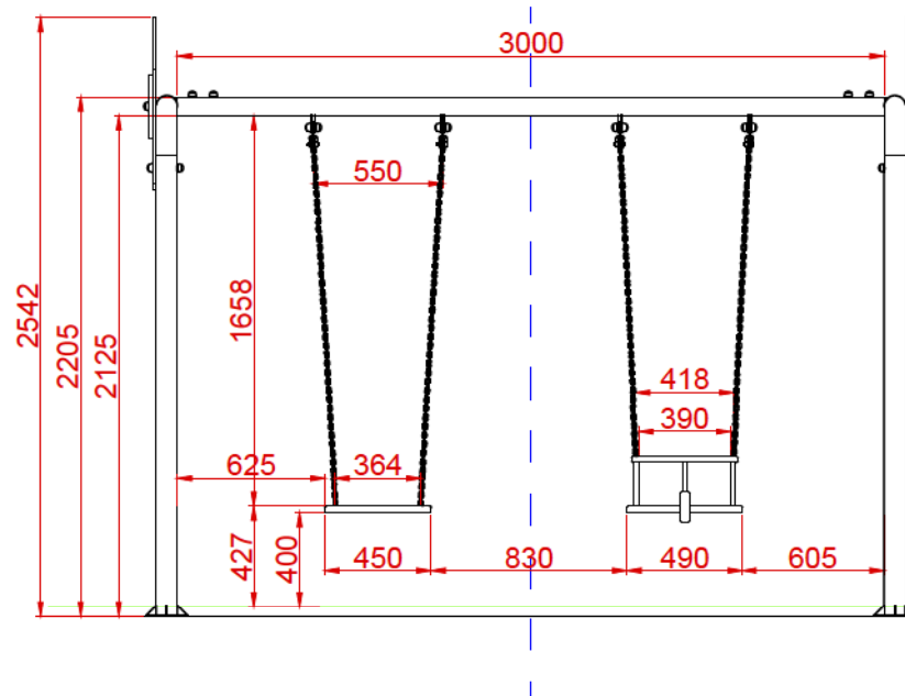
ALZADO
