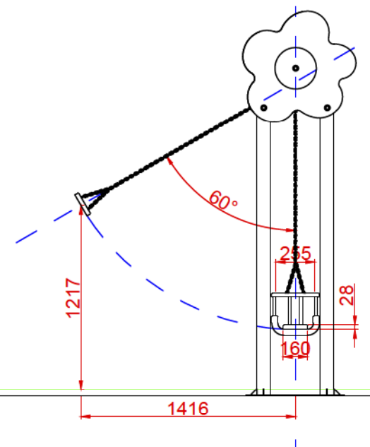
PERFIL
