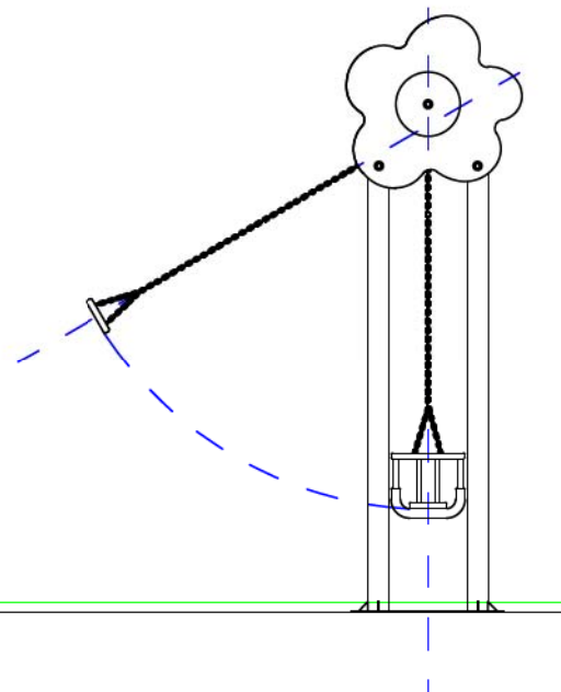
PERFIL
