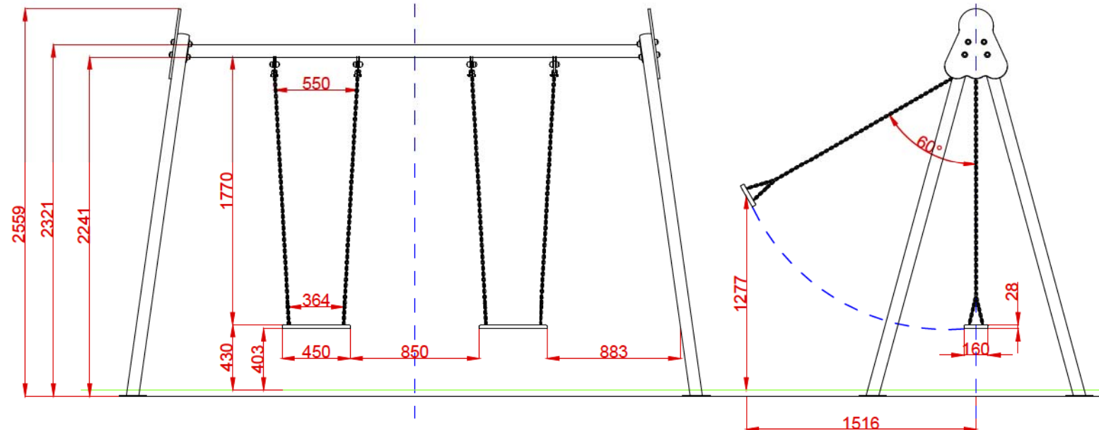
ALZADO
