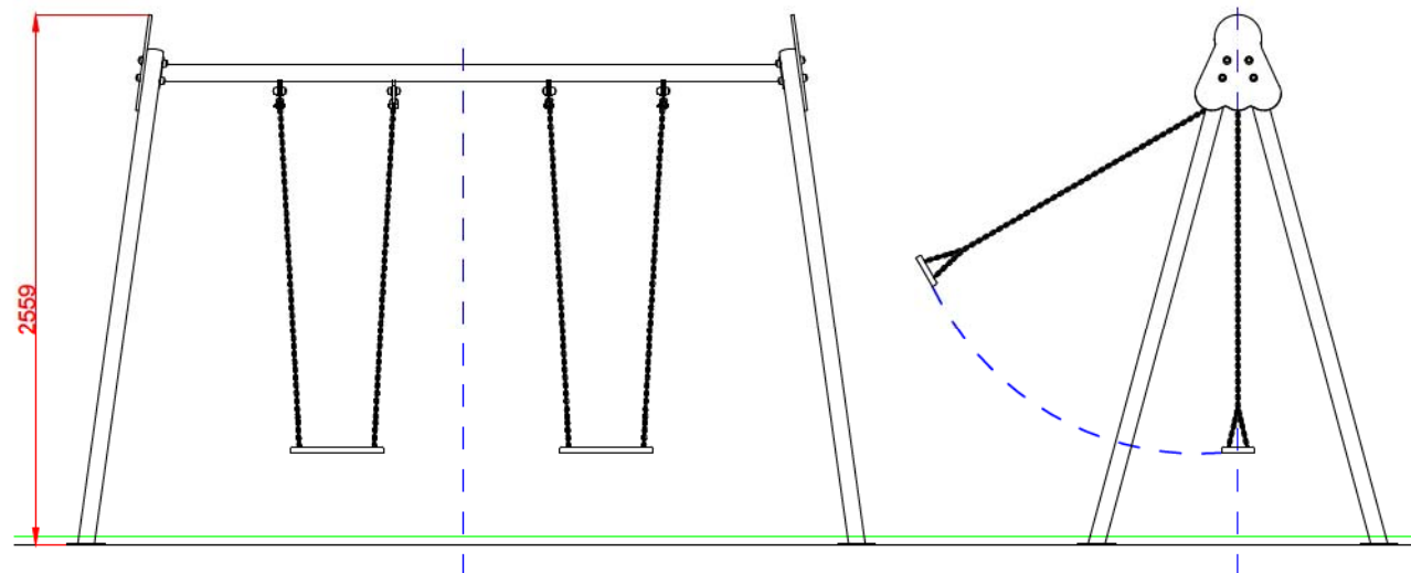
ALZADO
