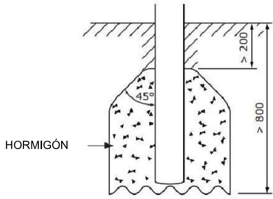
DETALLE CIMENTACIÓN
