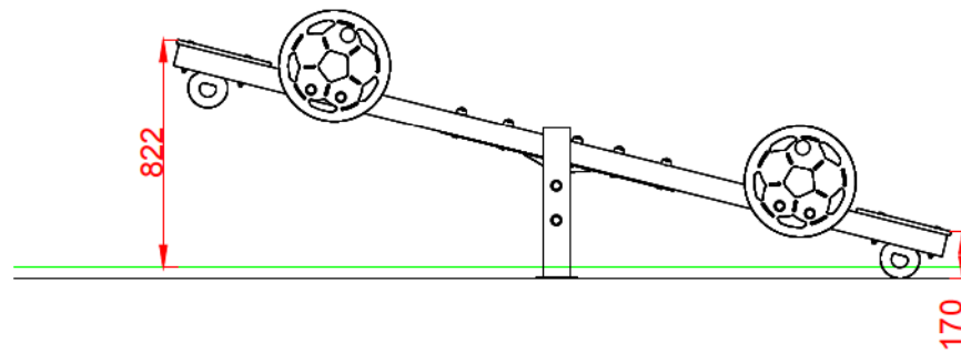
ALZADO
