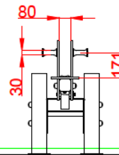
PERFIL
