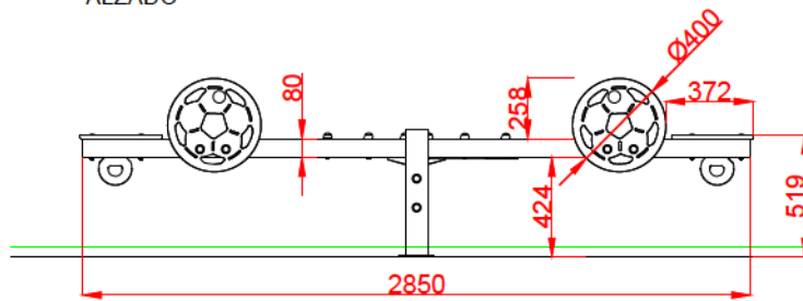
ALZADO
