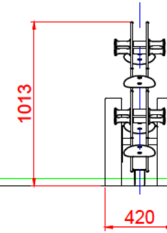
PERFIL
