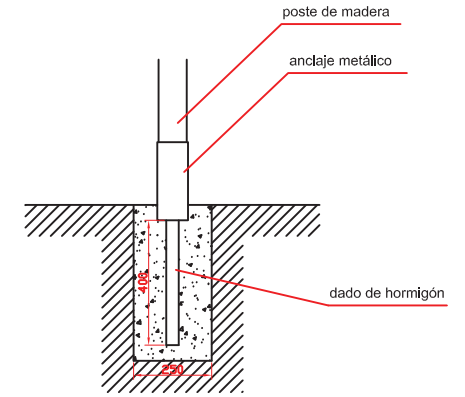
DETALLE DE CIMENTACIÓN E:2/1
