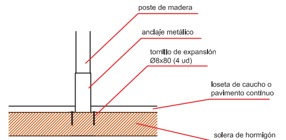
DETALLE DE ANCLAJES E:2/1
