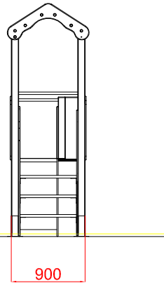
PERFIL DERECHO
