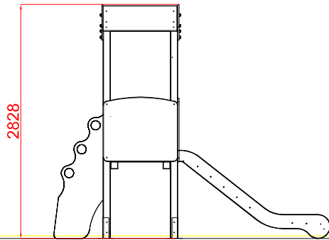
ALZADO
