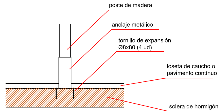
DETALLE DE ANCLAJES E:2/1
