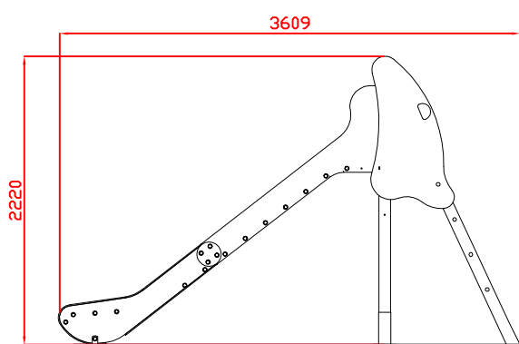
Alzado
