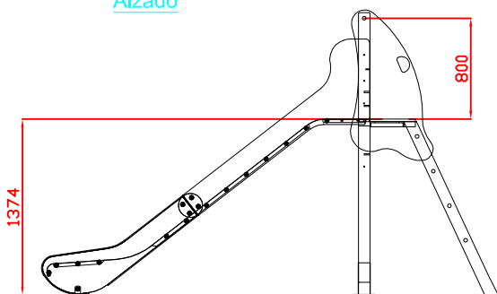
Alzado
