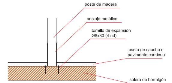
DETALLE DE ANCLAJE E:2/1
