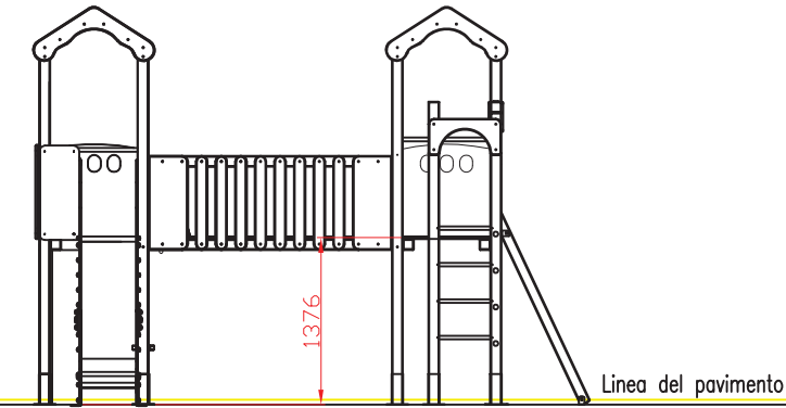
PERFIL DERECHO
