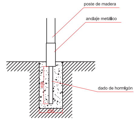
DETALLE DE CIMENTACIÓN E:2/1
