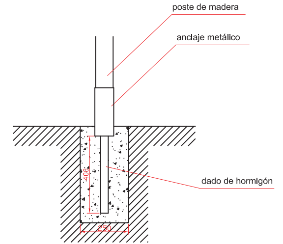
DETALLE DE CIMENTACIÓN E:2/1
