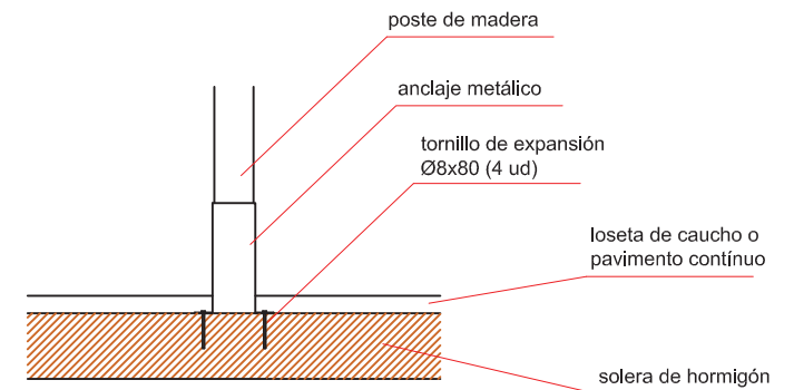
DETALLE DE ANCLAJES E:2/1
