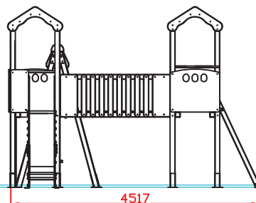
PERFIL IZQUIERDO
