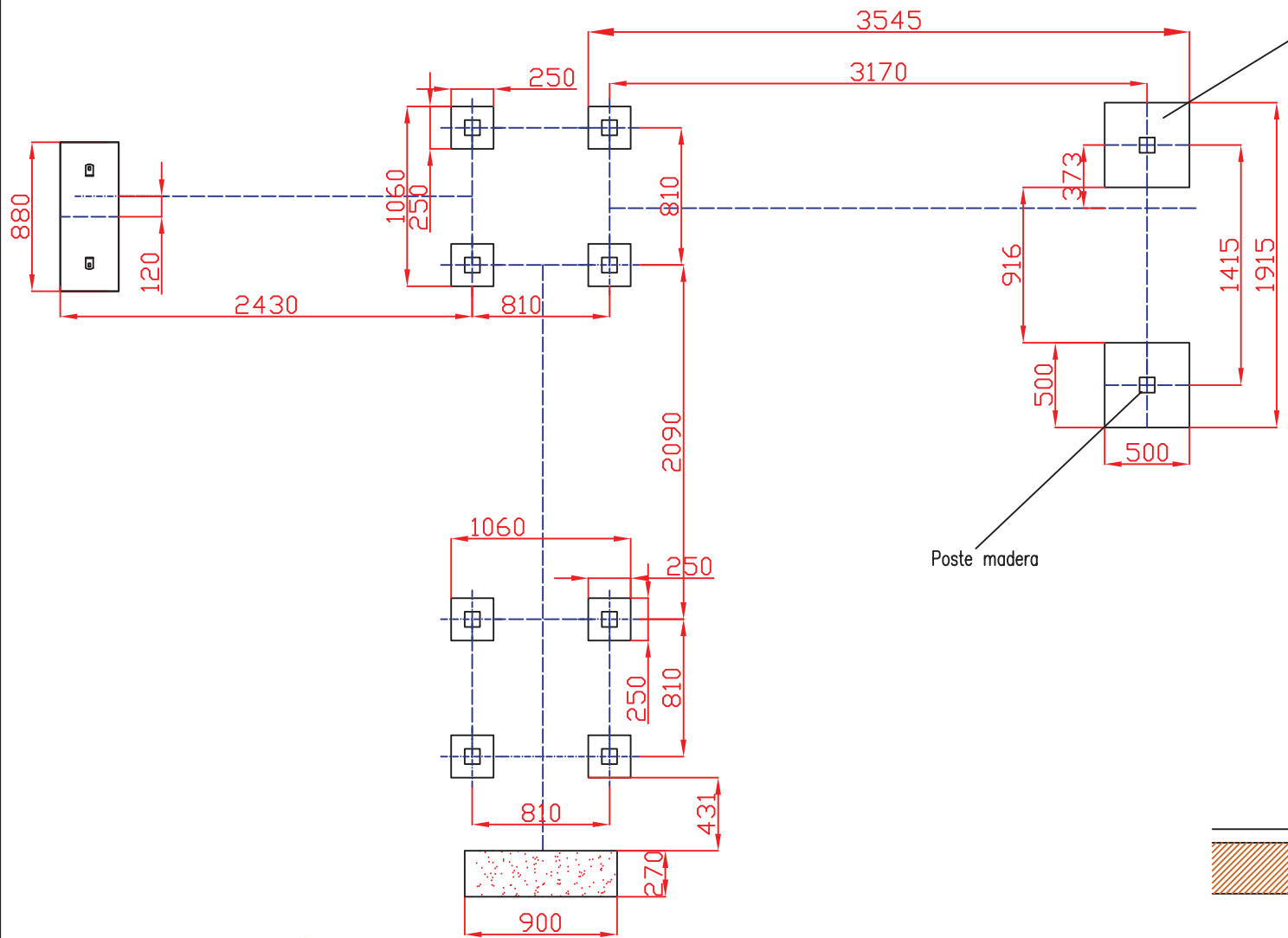
DETALLE DE ANCLAJES E:2/1
