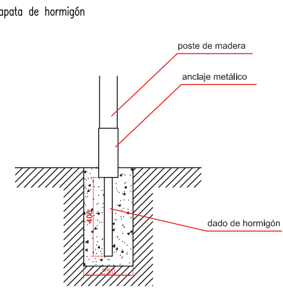
DETALLE DE CIMENTACIÓN E:2/1
