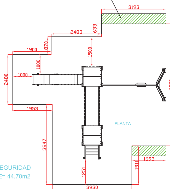
ZONA LIBRE DE OBSTÁCULOS
