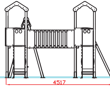
PERFIL IZQUIERDO
