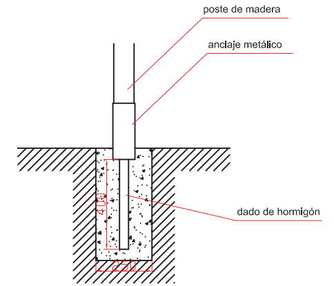
DETALLE DE CIMENTACIÓN
